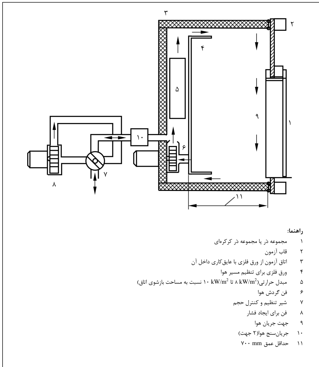
شکل ب-۱-نمایی از طرح اتاق آزمون
