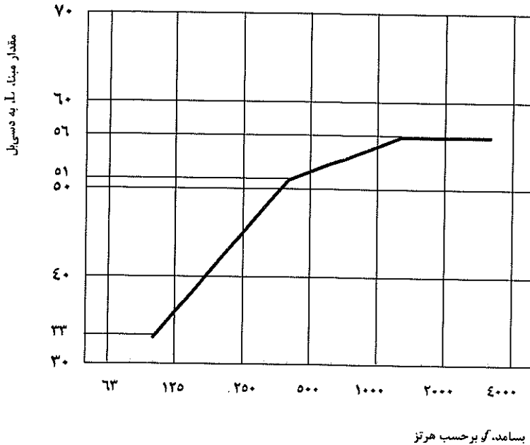
شکل ۱۸-۳-۴: نمودار مقادیر مینا برای صدای هواپرد، در بندهای یک‌سوم هنگامی
